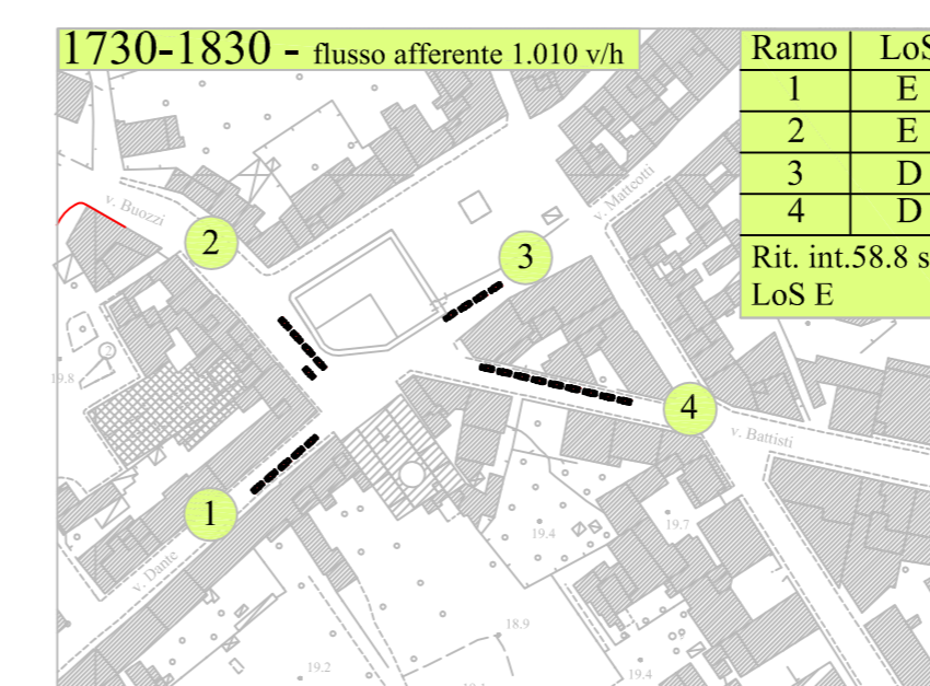
LoS e lunghezza code - Stato progetto Ciclo semaforico 110 sec.
