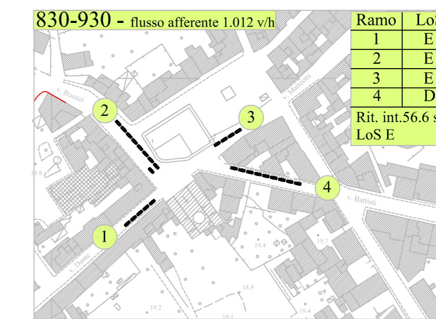
LoS e lunghezza code - Stato attuale Ciclo semaforico 153 sec
