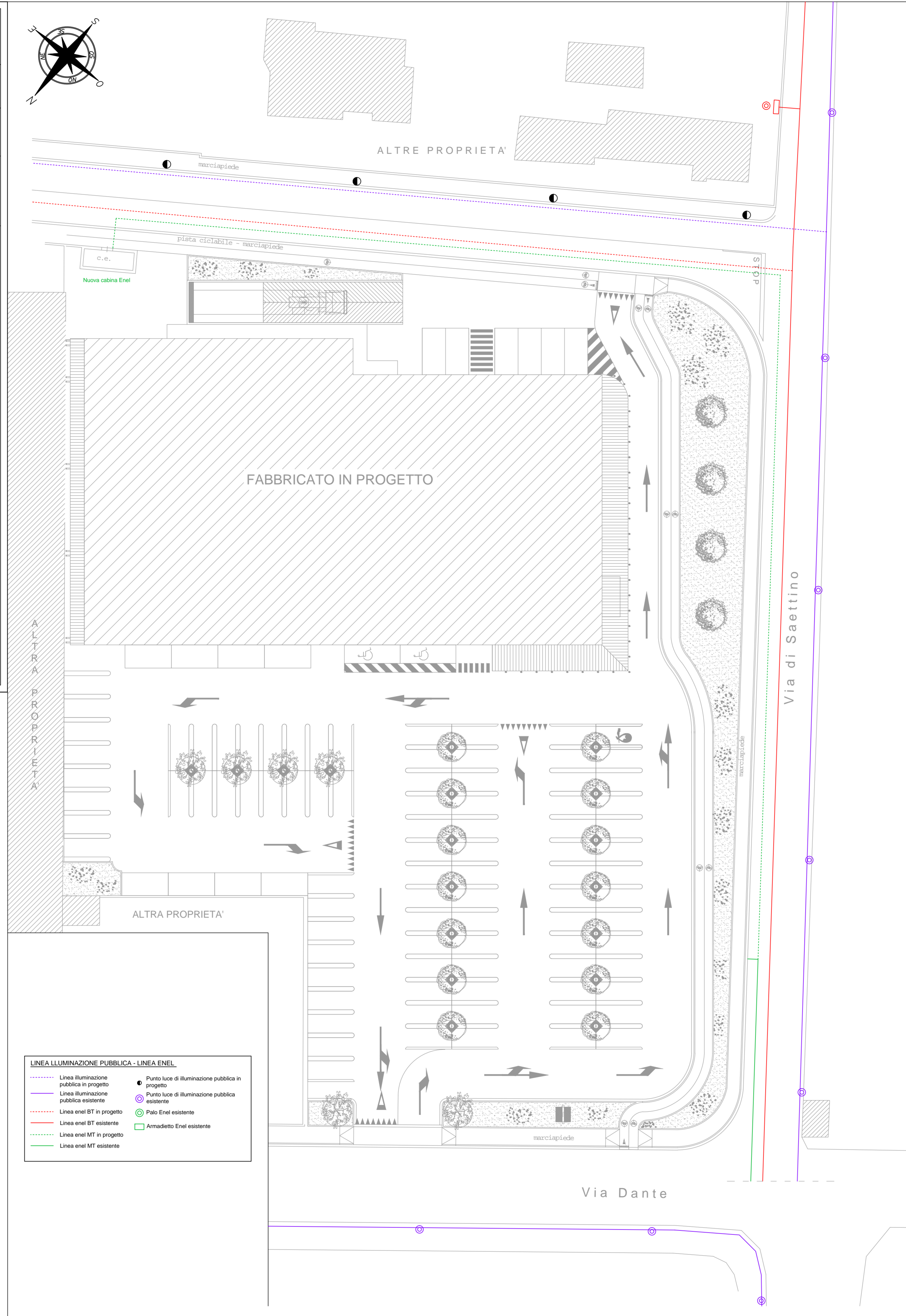
OPERE DI URBANIZZAZIONE: LINEA ILLUMINAZIONE PUBBLICA E FORNITURA ENERGIA ELETTRICA
